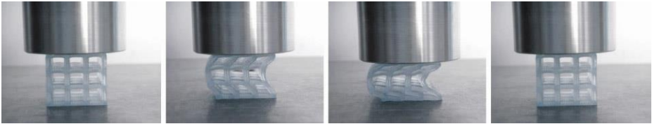
轻质网格结构决定了零件的压变特性
